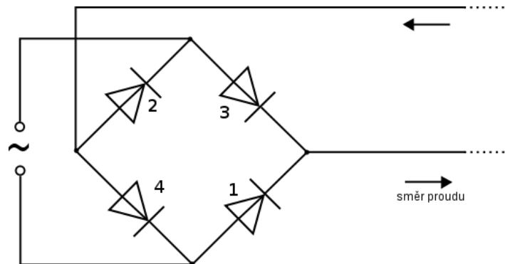
Graetzovo zapojení (dvoucestný usměrňovač)
